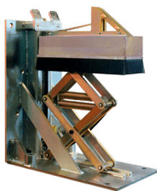
Retenedor de Barra Manual o Automática
