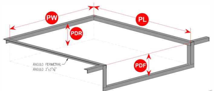
Isométrico Foso
