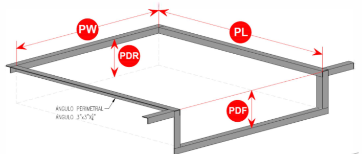
Isométrico Foso
